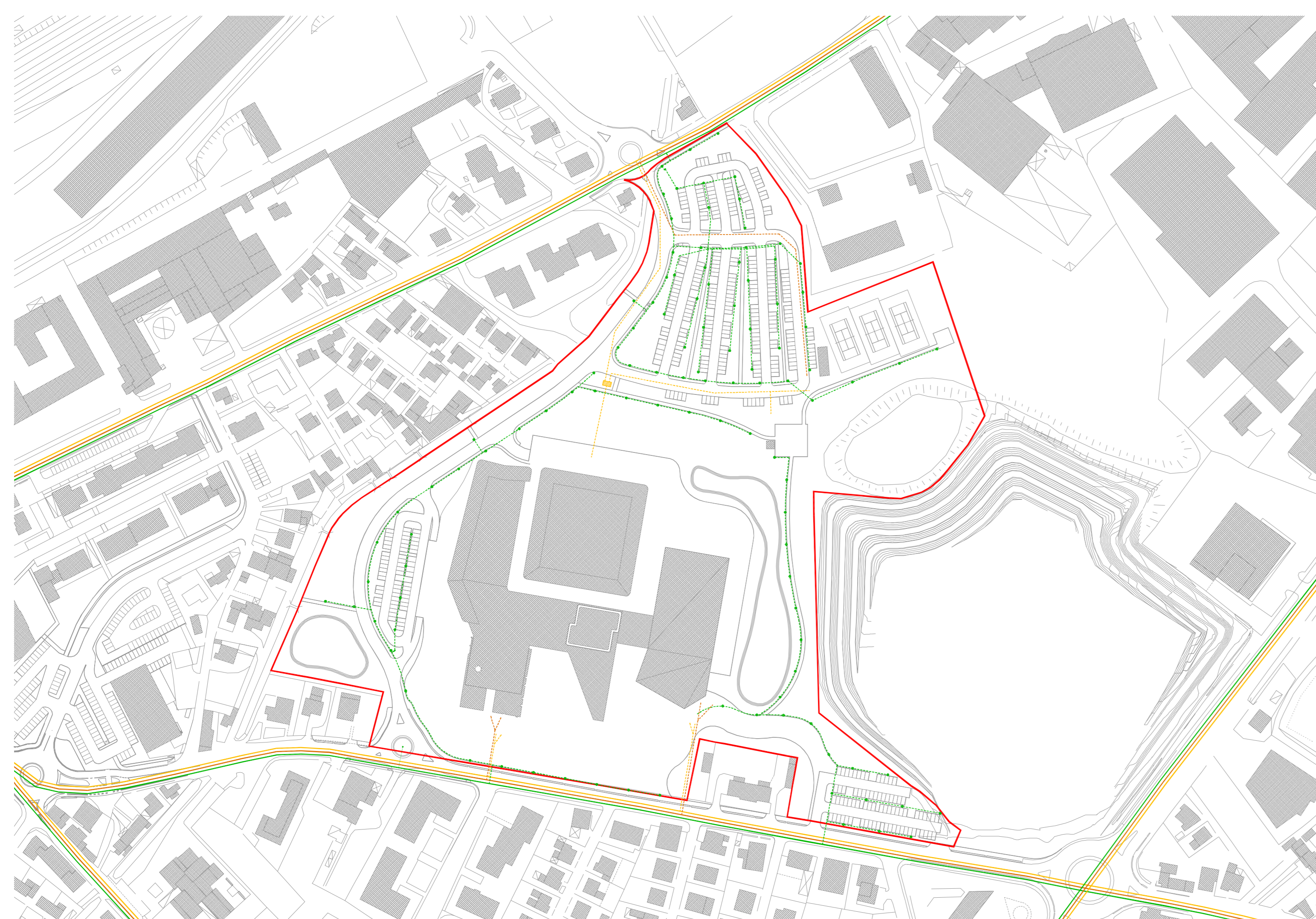
Planimetria rete illuminazione pubblica, Enel e Telecom
