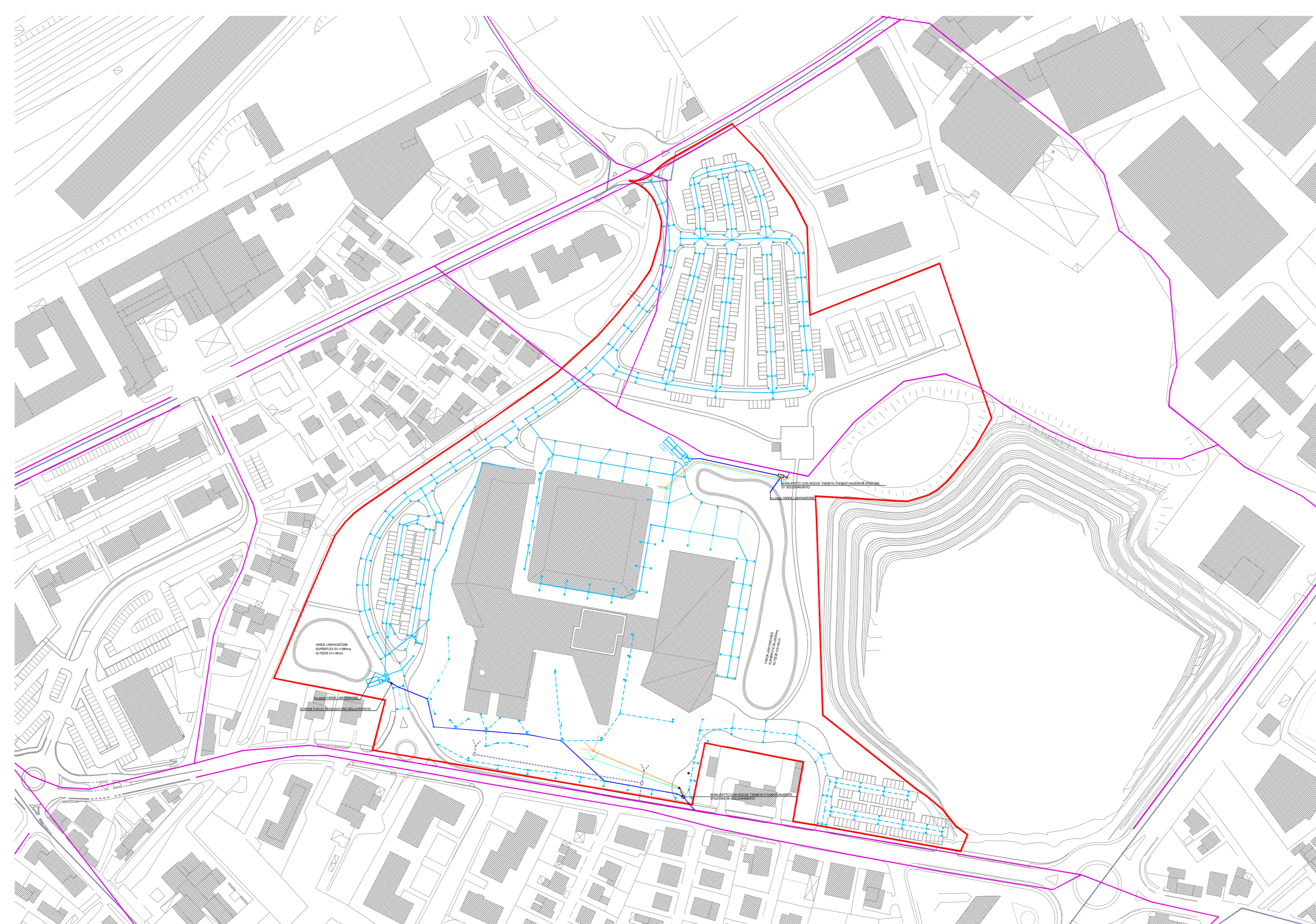
Planimetria rete acque meteoriche, acque miste ed acque nere
