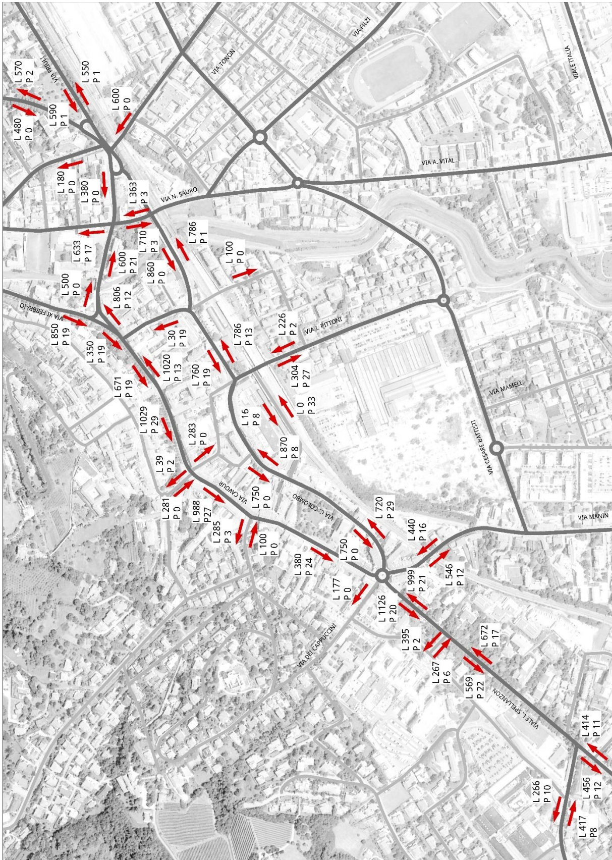
Figura 6: Centro - Flussi stato di progetto
