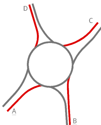
Figura 48: Schema rotatoria tra viale Italia e via San Giuseppe- stato di fatto e di progetto
