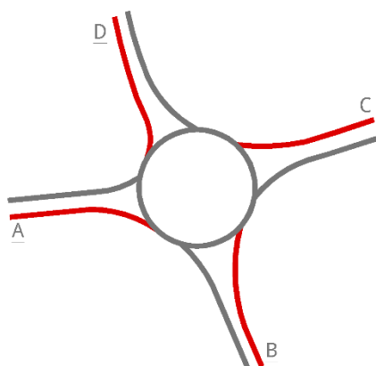
Figura 45: Schema rotatoria tra viale Italia e via Manin - stato di fatto e di progetto
