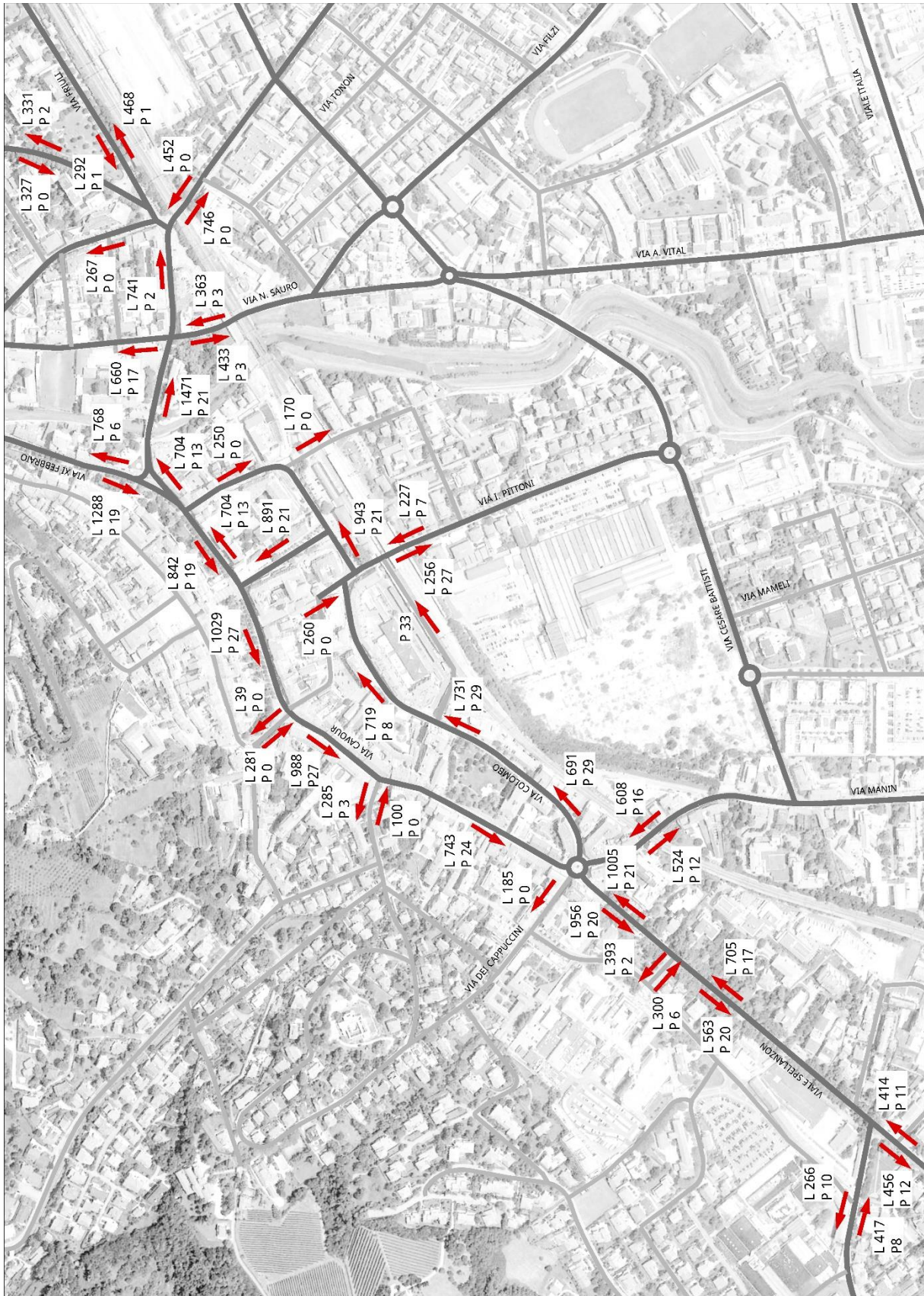
Figura 5: Centro - Flussi stato di fatto
