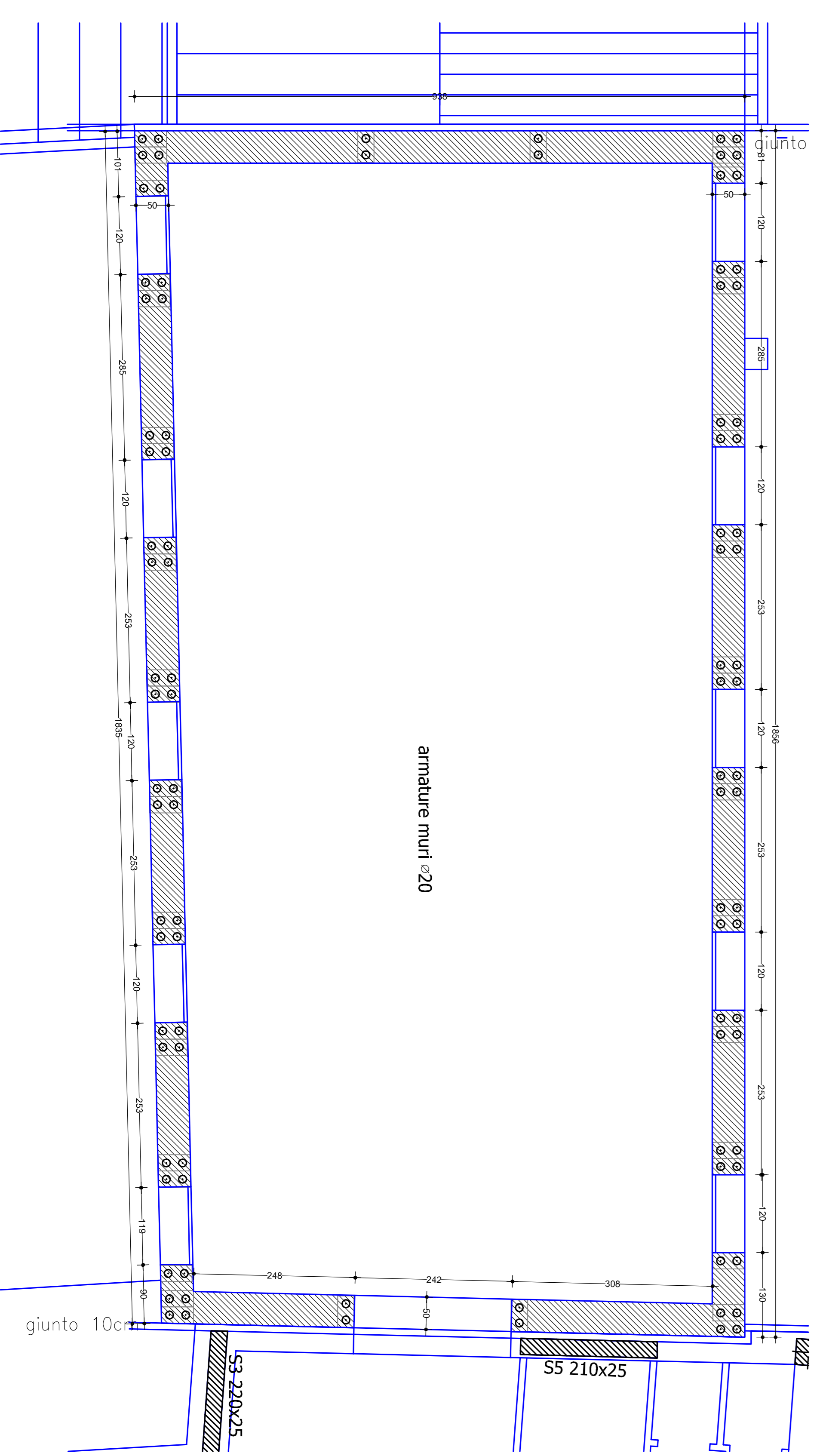
PIANTA MURATURE ARMATE AL PIANO SECONDO sc.1:150
